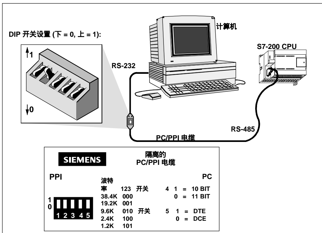
图 7 当数据从 RS-232 传送到 RS-485 口时，PC/PPI 电缆是发送模式。当数据从 RS-485 传送到 RS-232 口时，PC/PPI 电缆是接收模式。当检测到 RS-232 的发送线有字符时，电缆立即从接收模式切换到发送模式。当 RS-232 发送线处于闲置的时间超过电缆切换时间时，电缆又切换到接收模式。这个时间与电缆上的 DIP 开关设定的波特率选择有关。
